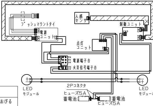
結線図
