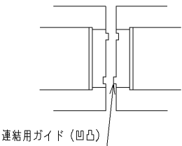
より確実に連結を行う場合は連結ガイドC-181（別売）をご使用ください。 直付け連結使用例
