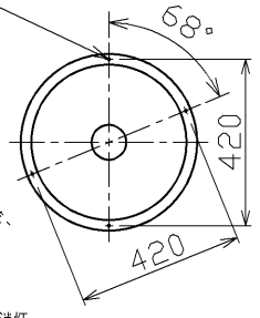
取付けピッチ寸法図 4-φ4.5木ねじ用K.○
