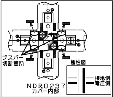
C, カバー内部図
