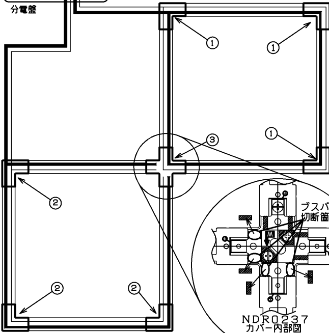
8の字施工 2回路分割時 バスバー切断箇所
