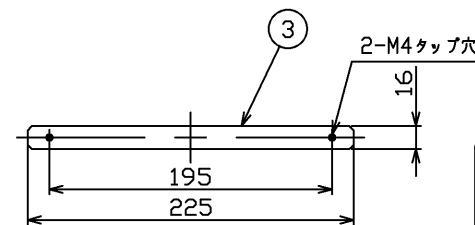
付属品 ガード取付金具
