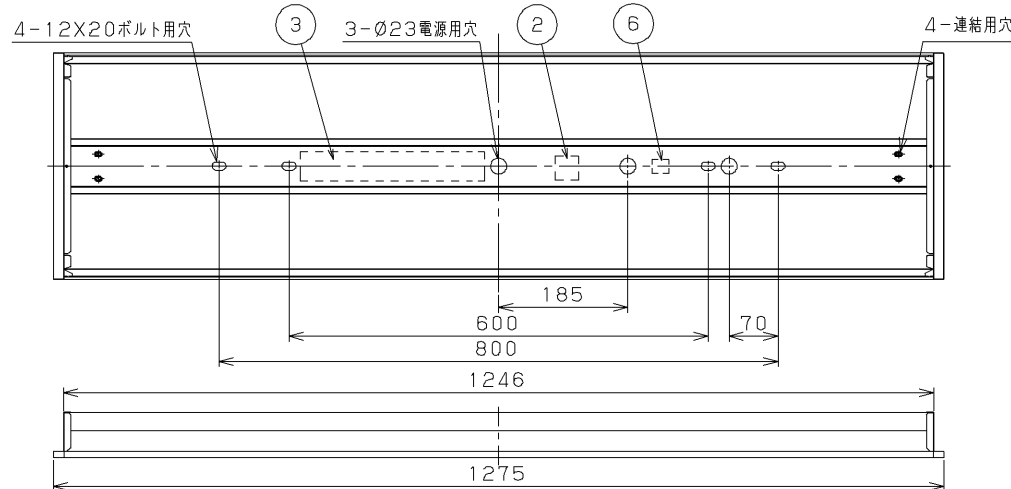
N連結の場合 1275×N-20 埋込み寸法
