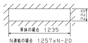
埋込み穴寸法
