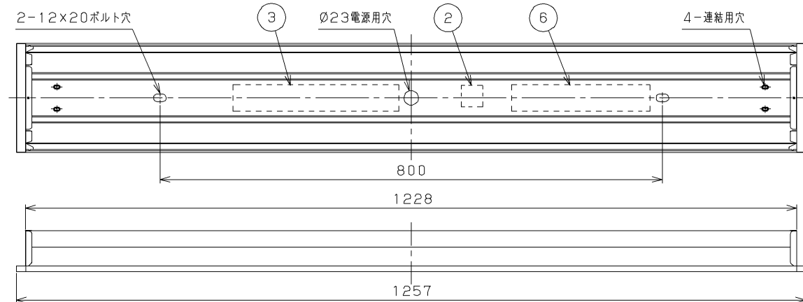
N連結の場合 1257×N-20 埋込み穴寸法
