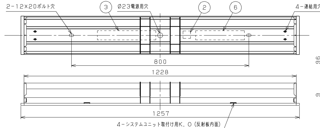
4-システムユニット取付け用K、O (反射板内面)
