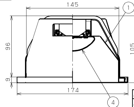
A寸法は25mmを越えないようにしてください。 取付ボルトを使用した場合の器具内寸法
