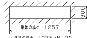
N連結の場合 1275×N-20 埋込み寸法
