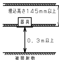
埋込み寸法
