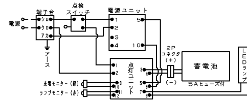
結線図
