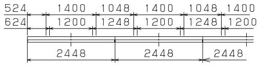
直付け連結使用例
