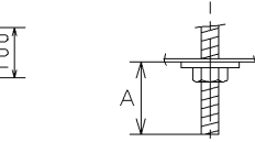
A寸法は25mmを超えないようにしてください。 取付けボルトを使用した場合の器具内寸法
