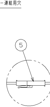
コネクタで電源ユニットとLEDバーを接続します。
