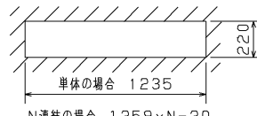
N連結の場合 1259×N-20 埋込み寸法
