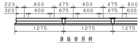
連結使用例
