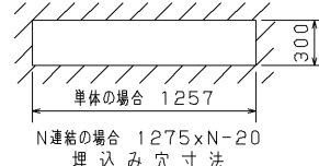
N連結の場合 1275×N-20 埋込み寸法
