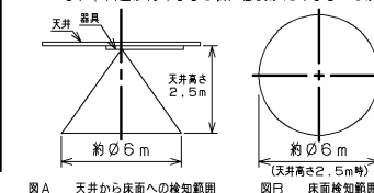
図A 天井から床面への検知範囲
