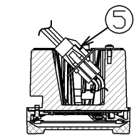
コネクタで電源ユニット LEDユニットを接続します。
