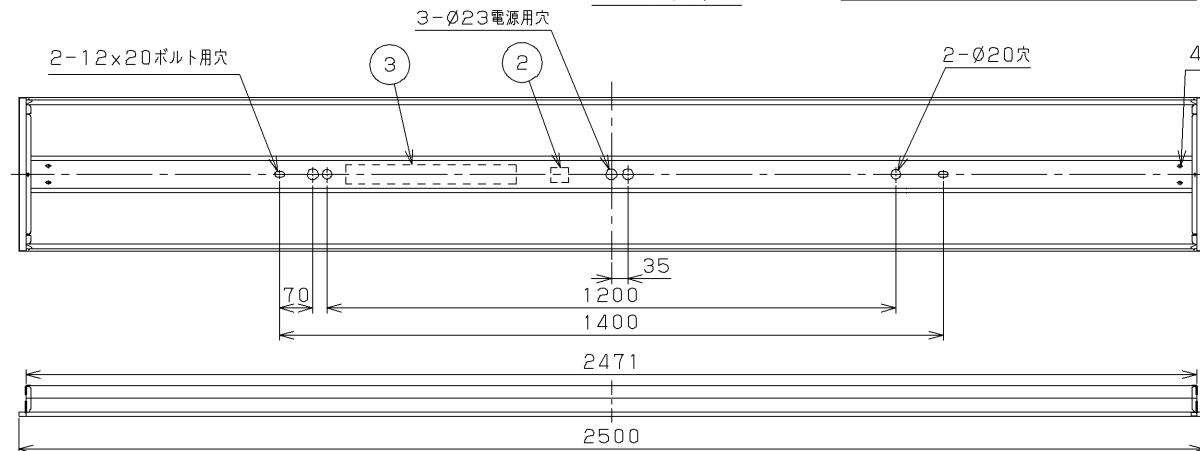
N連結の場合 2500×N-20 埋込み穴寸法
