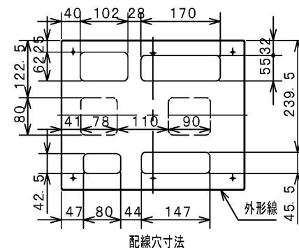
配線穴寸法
