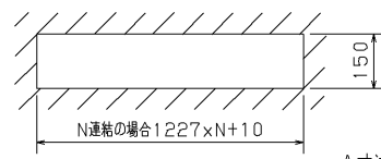
埋込み穴寸法
