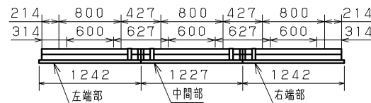
連結使用例
