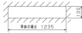
N連結の場合 1257×N-20 埋込み寸法
