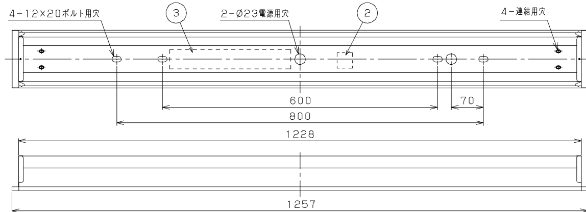
N連結の場合 1257×N-20 埋込み穴寸法
