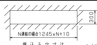
埋込み穴寸法
