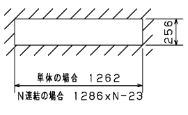
埋込穴寸法
