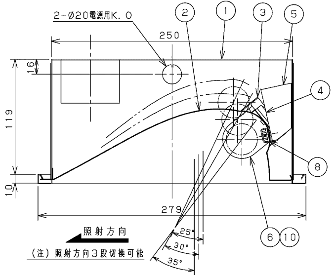
適合連結金具C-87
