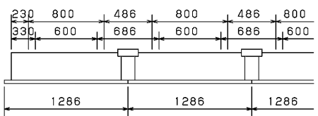
連結使用例
