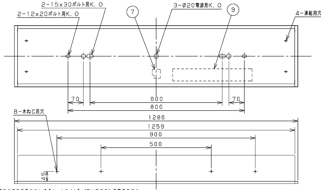
取付ボルトの器具内寸法
