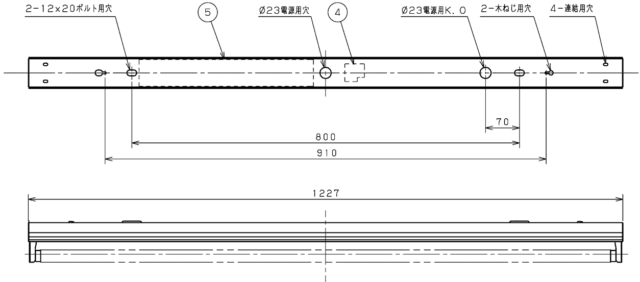
取付ボルトの器具内寸法
