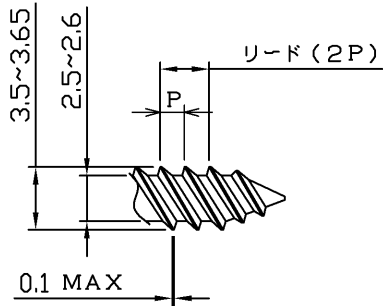
ねじ山部形状詳細 (ねじ山数: 18)
