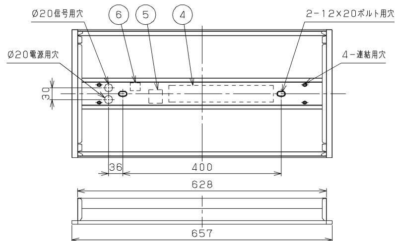
40タイプ器具N連結+20タイプ器具の場合 1275×N-20+657 埋込み穴寸法
