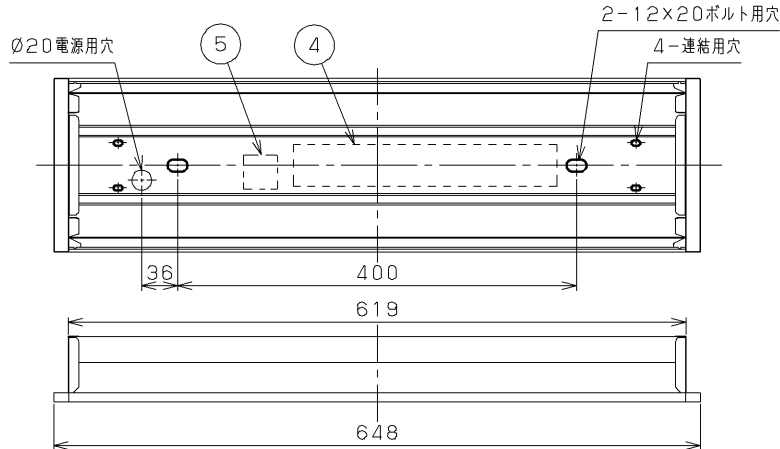
40タイプ器具N連結+20タイプ器具の場合 1257×N-20+648 埋込み穴寸法
