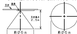
図A 天井から床面への検知範囲
