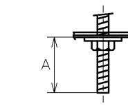
A寸法は20mmを超えないようにしてください。 取付けボルトを使用した場合の器具内寸法
