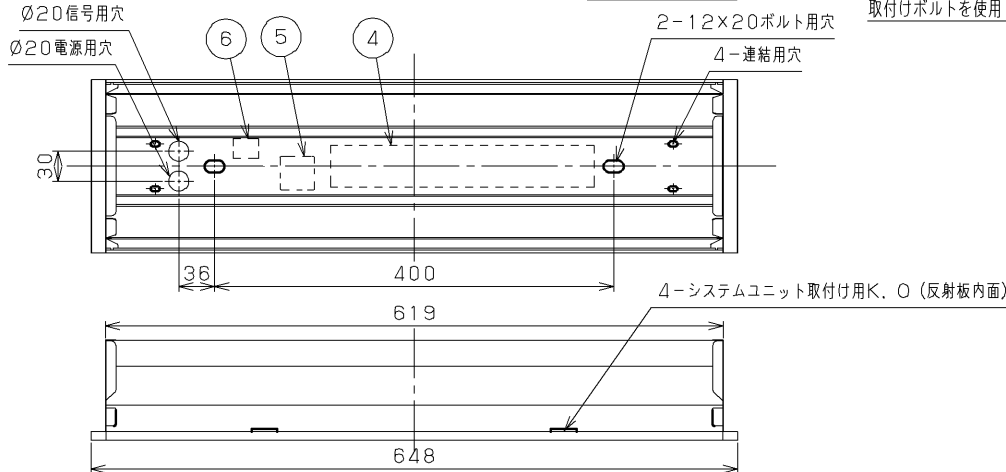
40タイプ器具N連結+20タイプ器具の場合 1257 x N - 20 + 648
