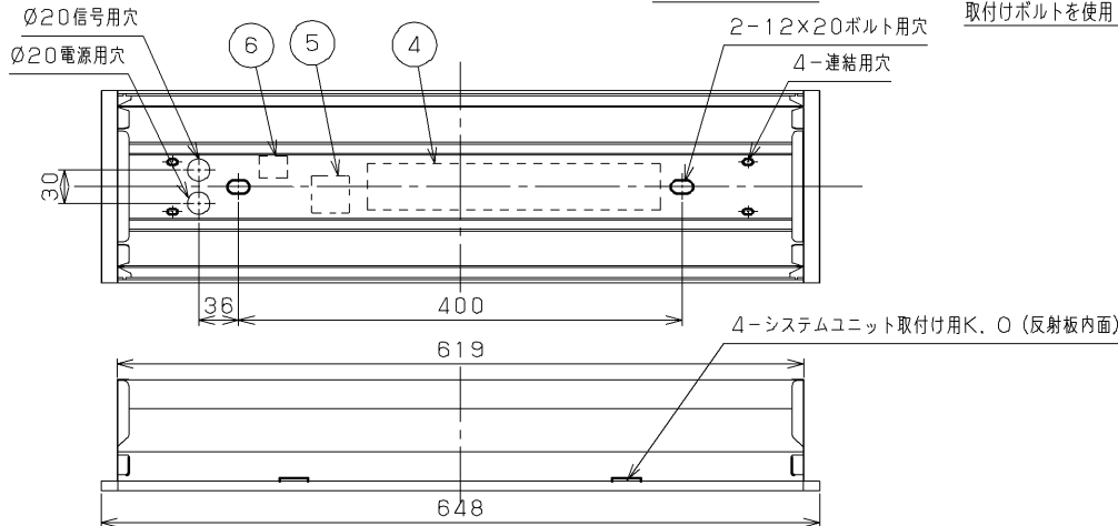
40タイプ器具N連結+20タイプ器具の場合 1257×N-20+648 埋込み穴寸法
