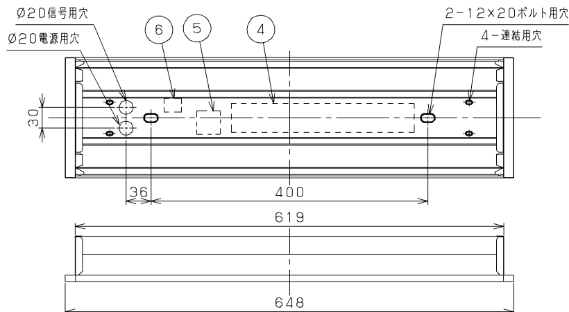
40タイプ器具N連結+20タイプ器具の場合 1257 \times N - 20 + 648 埋込み穴寸法
