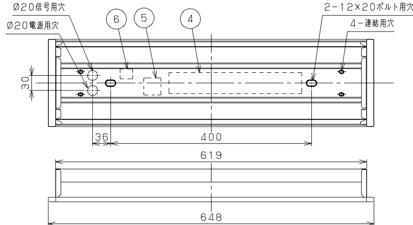
40タイプ器具N連結+20タイプ器具の場合 1257×N-20+648 埋込み穴寸法
