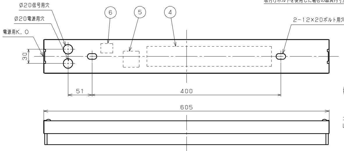
直付け連結使用例
