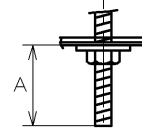
A寸法は20mmを超えないようにしてください。 取付けボルトを使用した場合の器具内寸法
