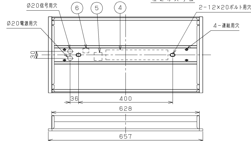
埋込み寸法
