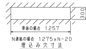
N連結の場合 1275×N-20 埋込み穴寸法
