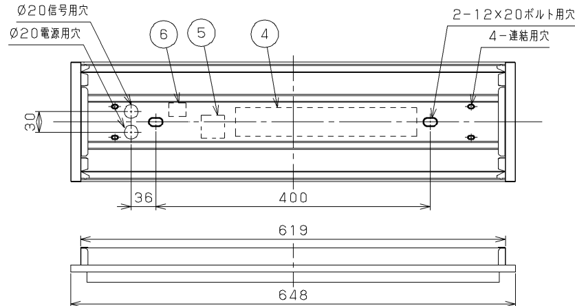
40タイプ器具N連結+20タイプ器具の場合 1257×N+20+648 埋込み穴寸法
