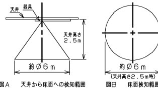
図A 天井から床面への検知範囲
