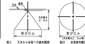
図A 天井から床面への検知範囲
