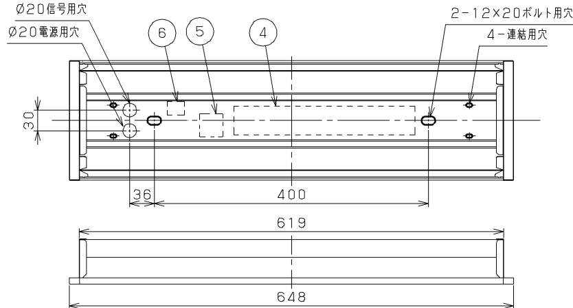
40タイプ器具N連結+20タイプ器具の場合 1257×N-20+648 埋込み寸法
