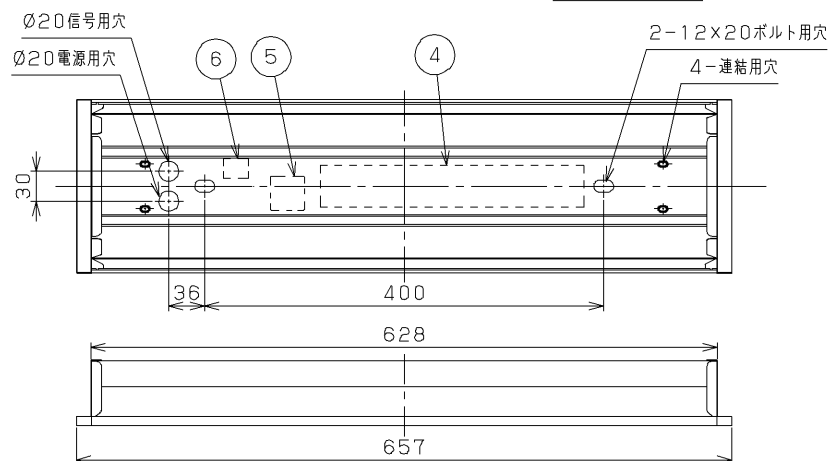
40タイプ器具N連結+20タイプ器具の場合 1275 \times N - 20 + 657 埋込み穴寸法
