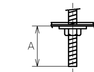
A寸法は20mmを超えないようにしてください。 取付けボルトを使用した場合の器具内寸法
