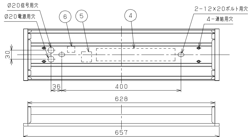
40タイプ器具N連結+20タイプ器具の場合 1275×N+20+657 埋込み寸法
