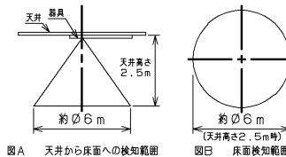
図A 天井から床面への検知範囲
