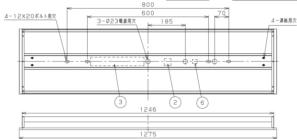
N連結の場合 1275×N-20 埋込み寸法
