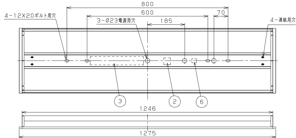
N連結の場合 1275mm x N-20 埋込み寸法
